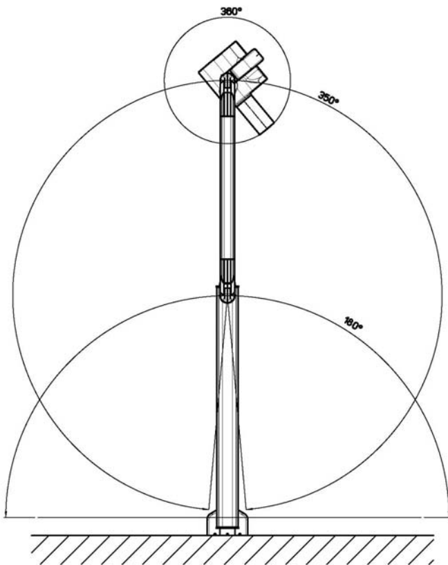
Fig. 3 – Maximum Reach (Extension) – Top view. Estensione massima – Vista dall'alto.
