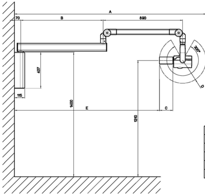
Fig. 2 – Maximum Reach (Extension) – For different brackets see table above. Estensione massima – Le misure delle diverse mensole sono riportate in tabella.
